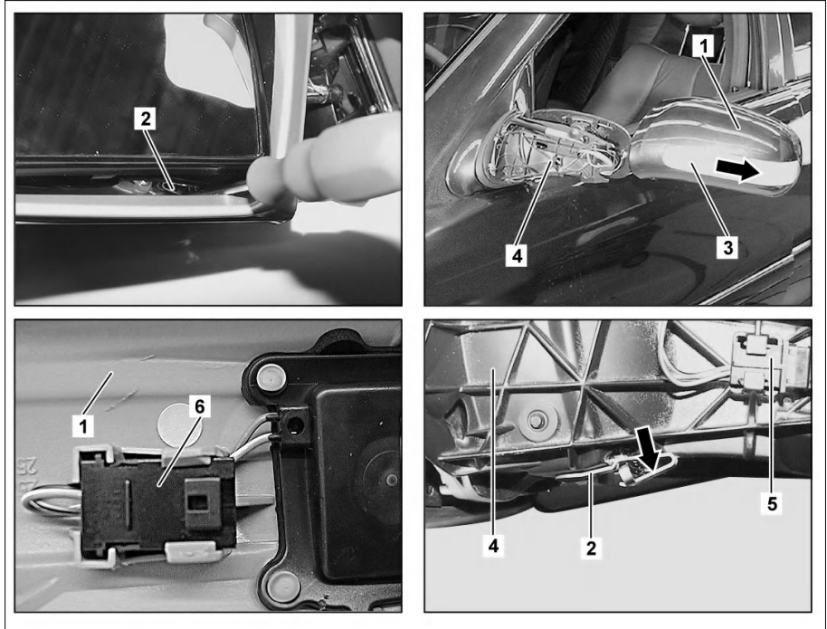
P88.70-2033-06
