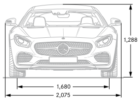
Mercedes-AMG GT/S Coupé
