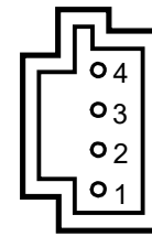
conn. I2
