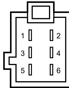
conn. M1
